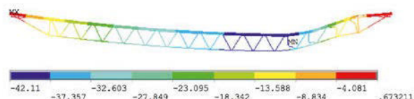
Diese Illustration aus dem NIST-Bericht [NCSTAR 1-6C, S. 77 (pdf: 125) – A. d. Ü.] zeigt das Durchhängen eines der fachwerkartigen Deckenträger um etwa 1 m.
